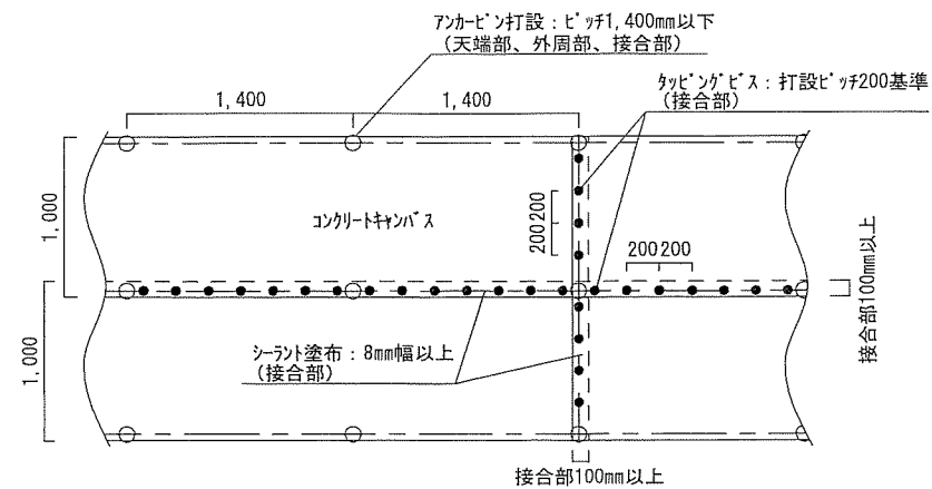
C 施工詳細 S=N/S
