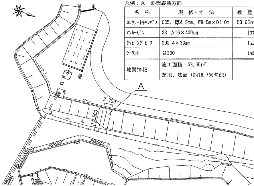
A 施工箇所 S=1/2,000
