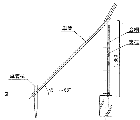
金網柵補強図 S=N/S
