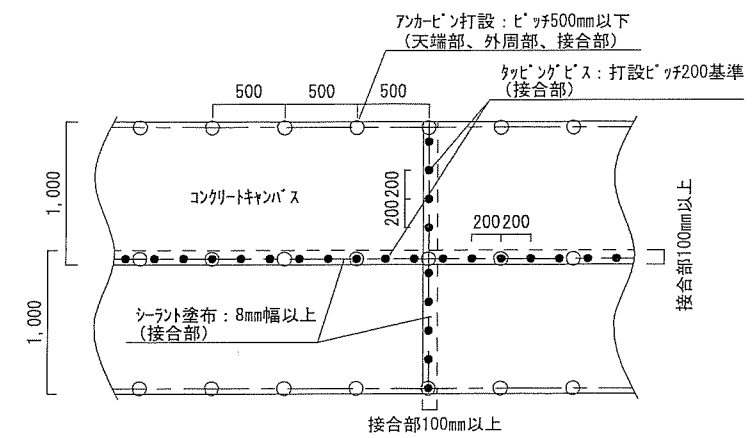
B 施工詳細 S=N/S
