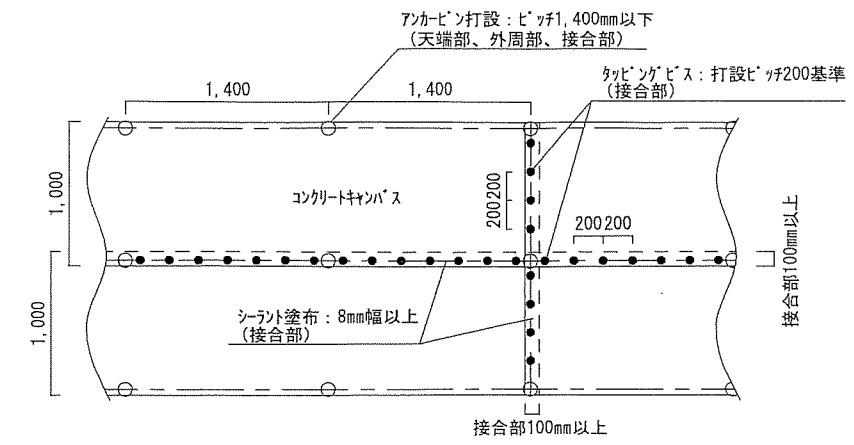
A 施工詳細 S=N/S
